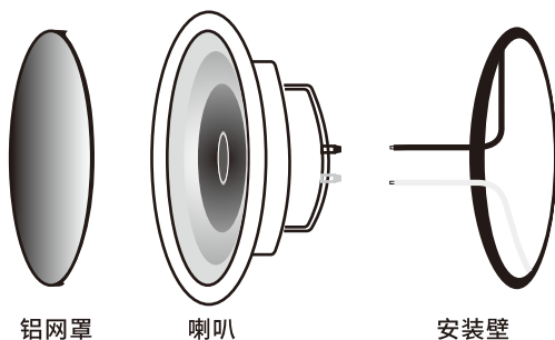
安装示意图
